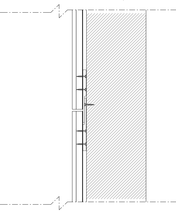
▼ Sezione orizzontale
