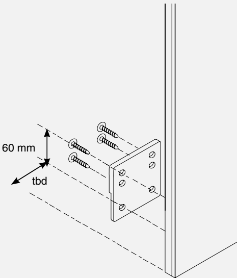
4 - EasyPlate - Parte bassa del pannello
