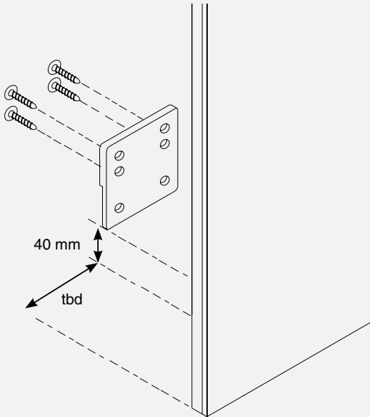
2 - EasyPlate - Pannello di base
